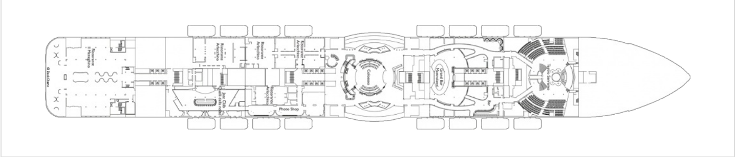
Палуба 6
