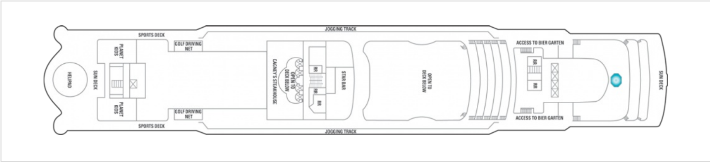
Палуба 14
