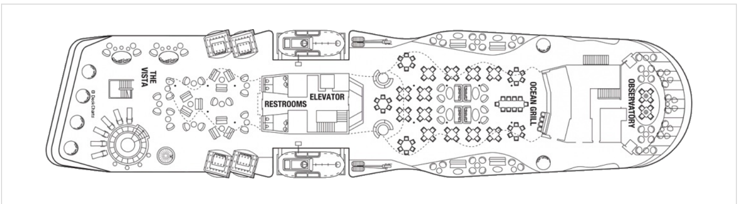
Палуба 7
