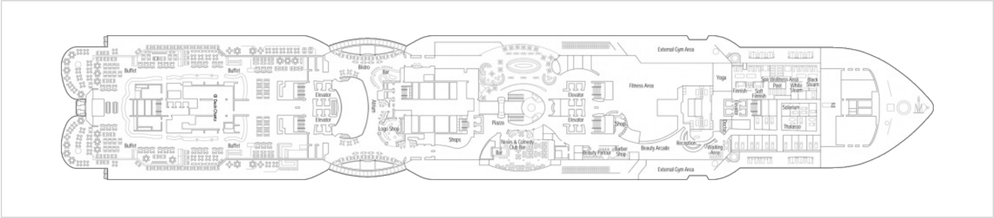
Палуба 9
