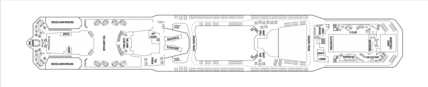
Палуба 15
