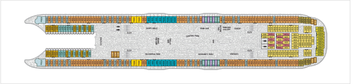
Палуба 8
