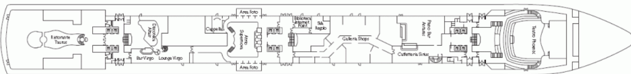
Палуба 3 - Ambra
